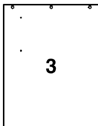
3 Lateral derecho 710x550 mm 53114/361314
